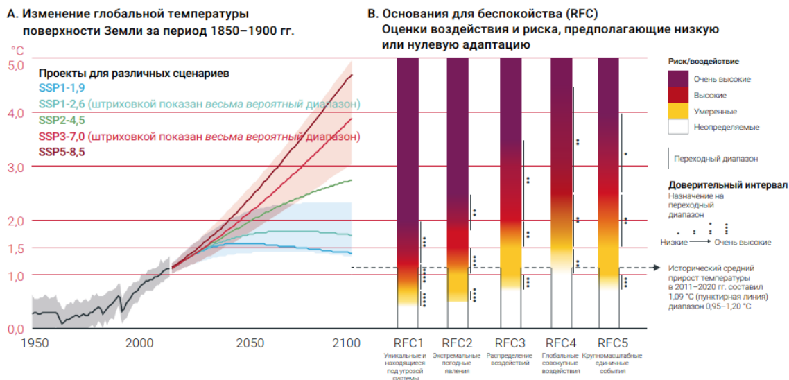
Рисунок 2. Прогнозы глобальных сценариев изменения климата
